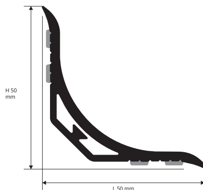
PSA 50-... / PSA 50-... A scala 1:1
